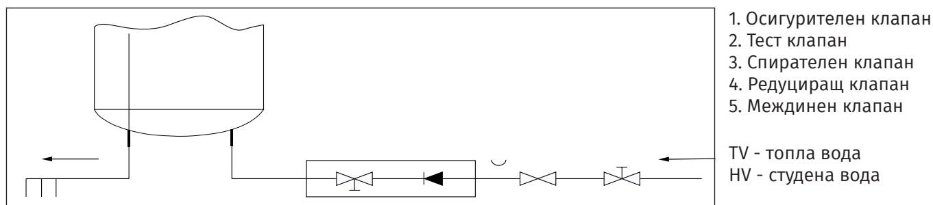
Схема 2 - захранване на бойлера без монтаж на разширителен съд и връзка със сифон
